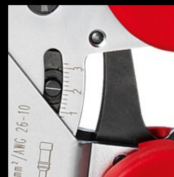
Anzeigebereich, Zwangssperre
